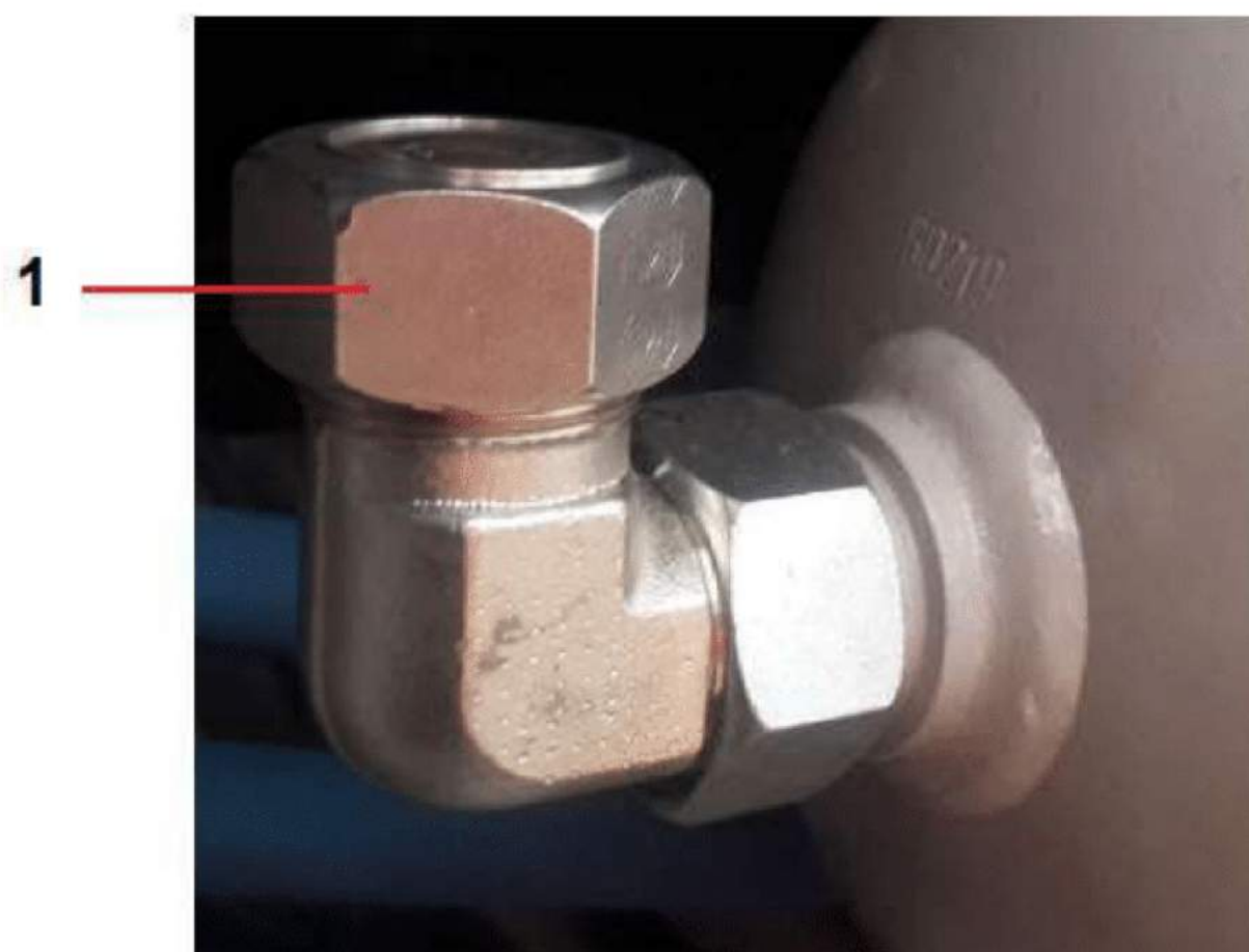
Рисунок-7 Заправка сепараторного бака маслом (1)
