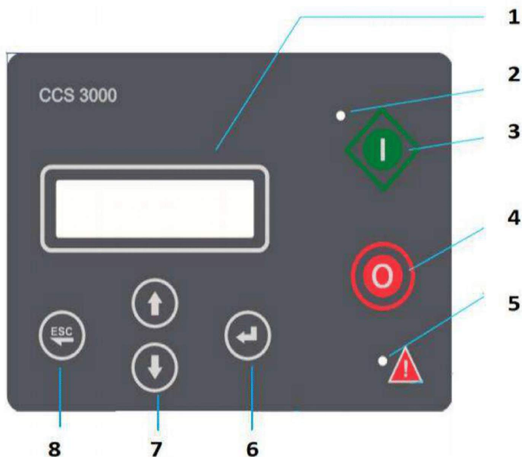
Рисунок 4 Панель управления CCS3000
