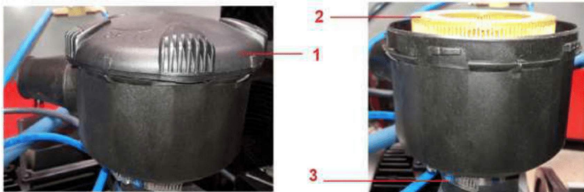
Рисунок-11 Замена элемента воздушного фильтра
