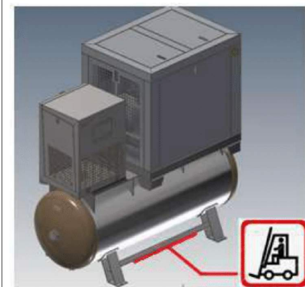
Рисунок-5b Точка подъема вилочного погрузчика
