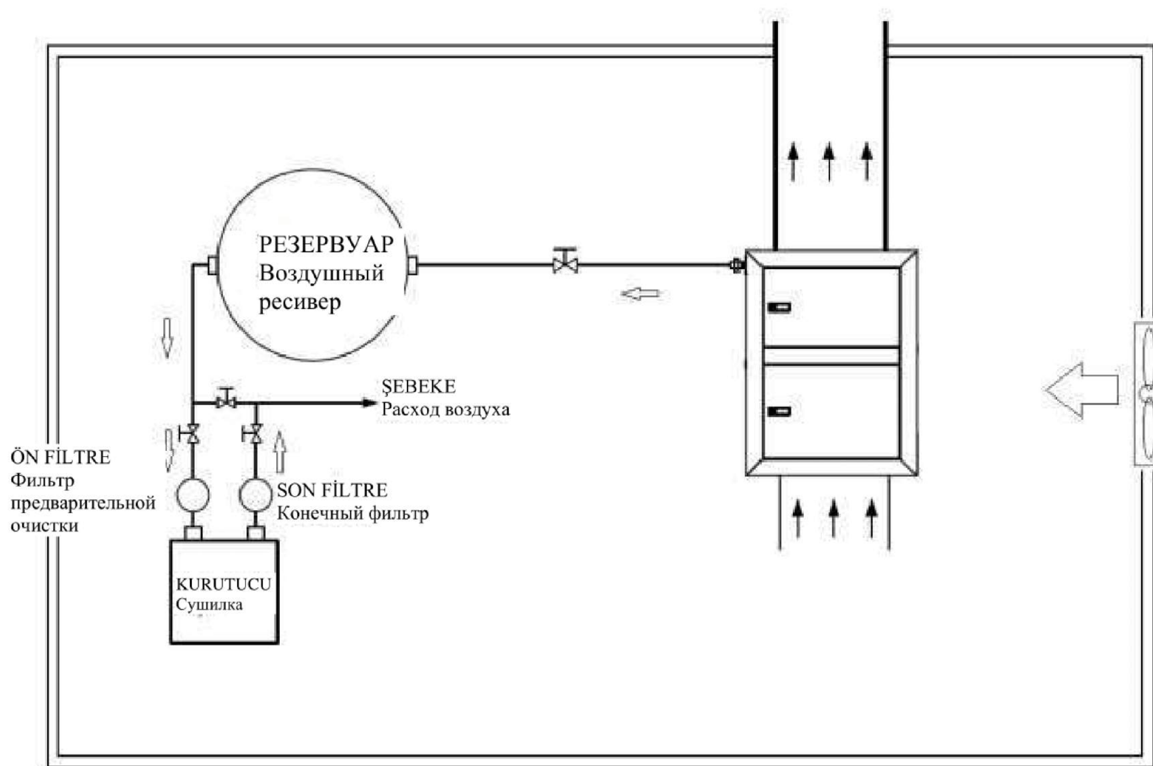
Схема-3 Пример планировки компрессорной
