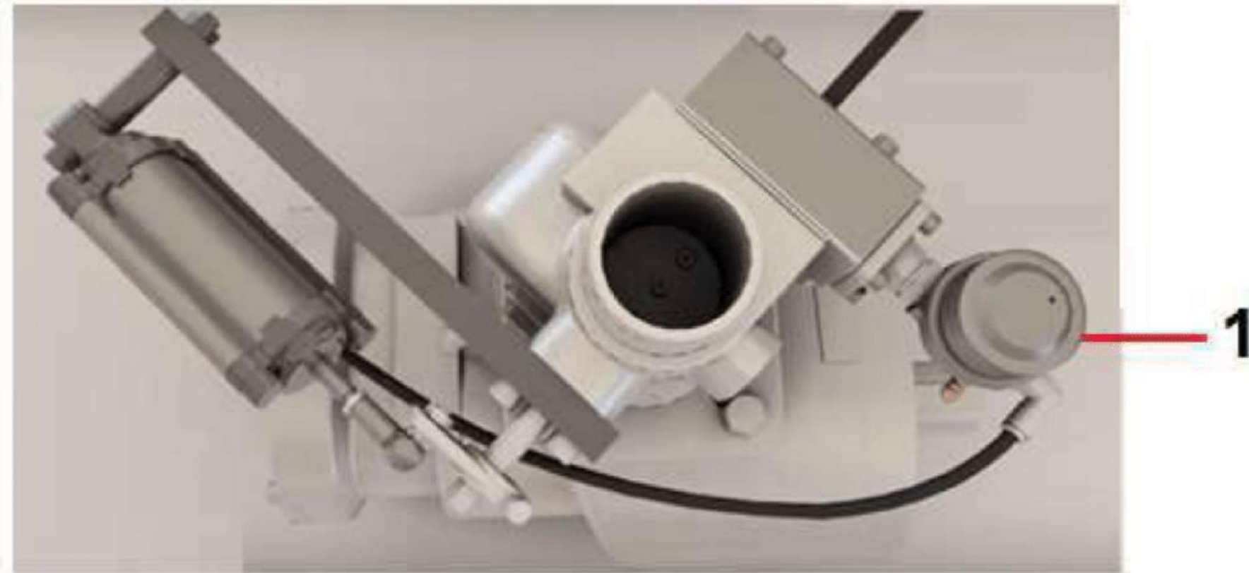
Рис. 3 Пропорциональный распределитель (1) в системе управления всасыванием
