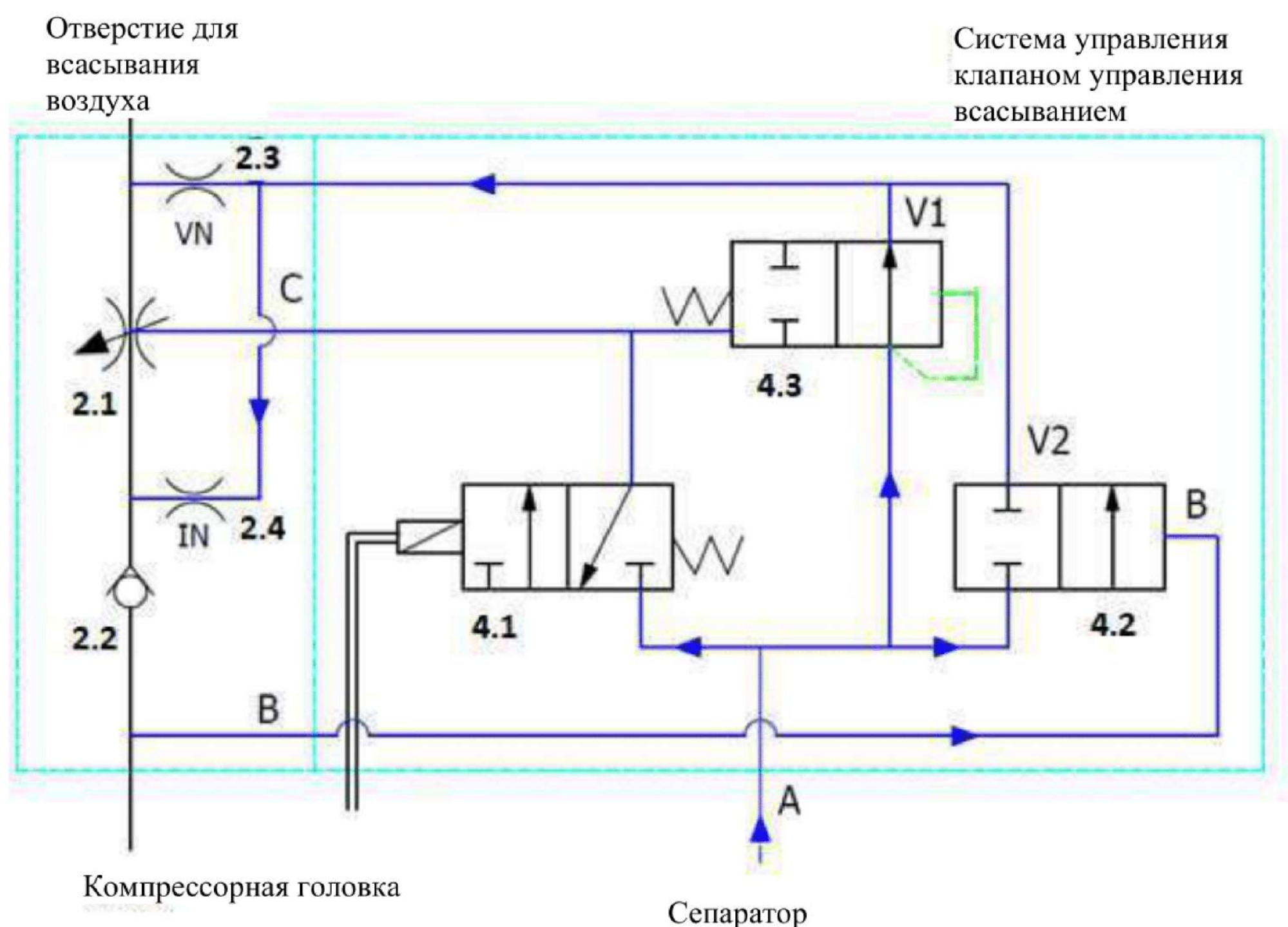
Схема 1.1 Система управления с клапаном управления всасыванием НАКГ
