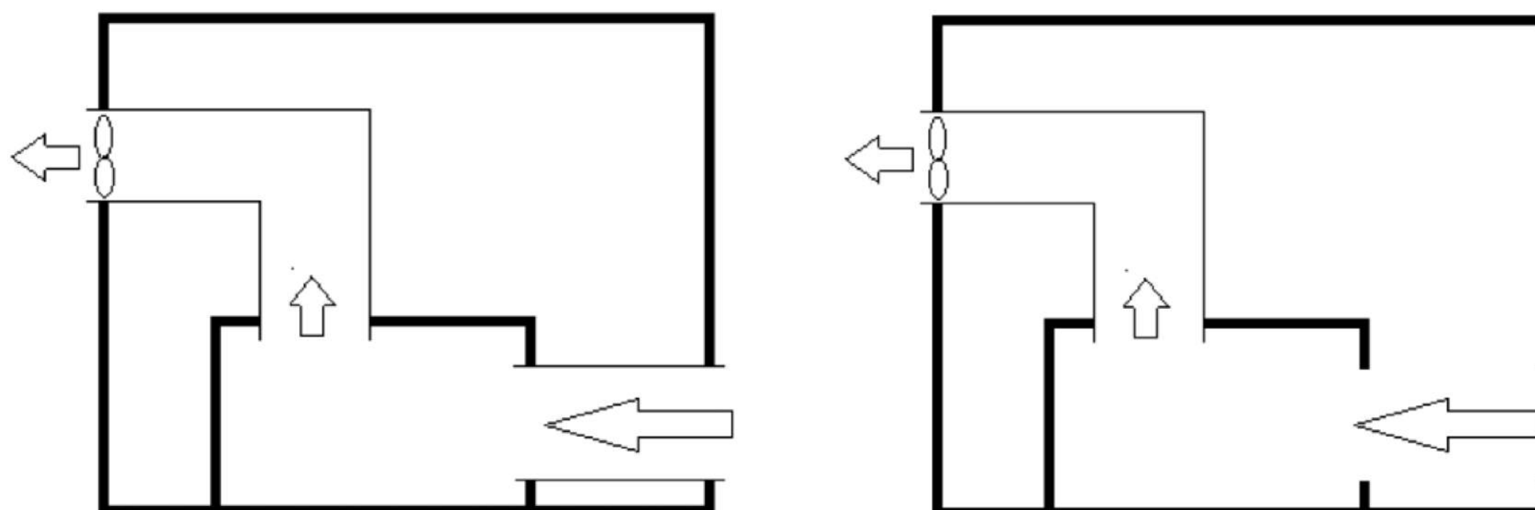
Схема -2 Примеры вентиляции компрессорной
